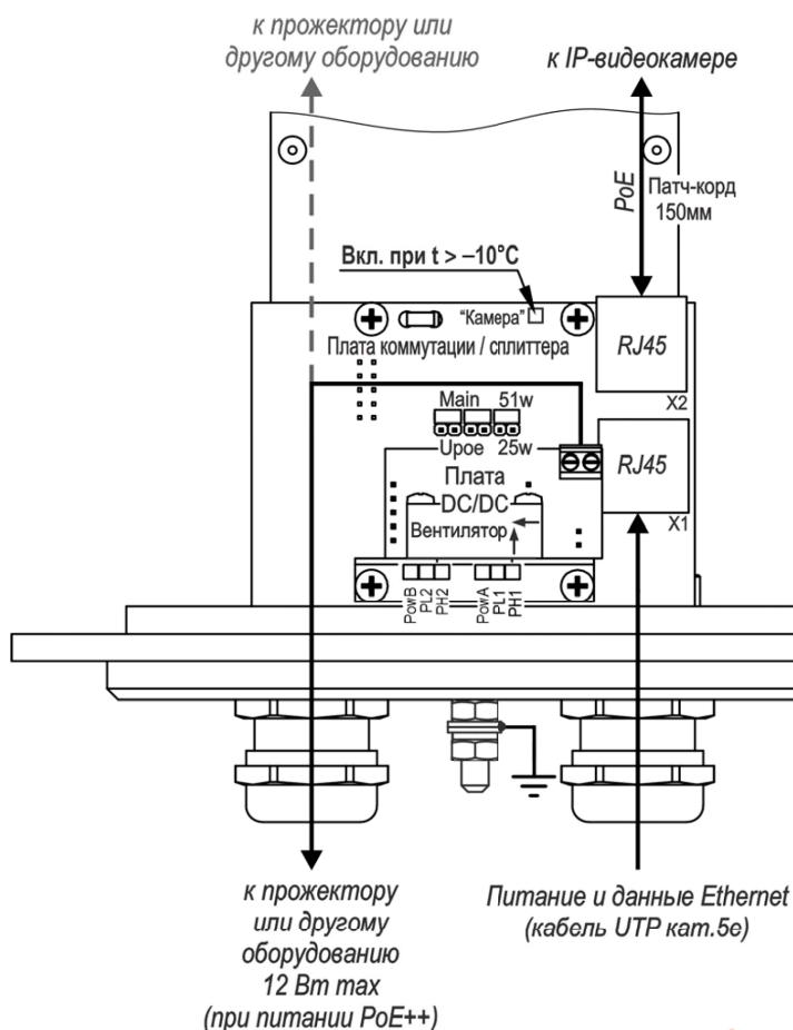
Рисунок 4 – Подключение ТГБ-11-Рое++
