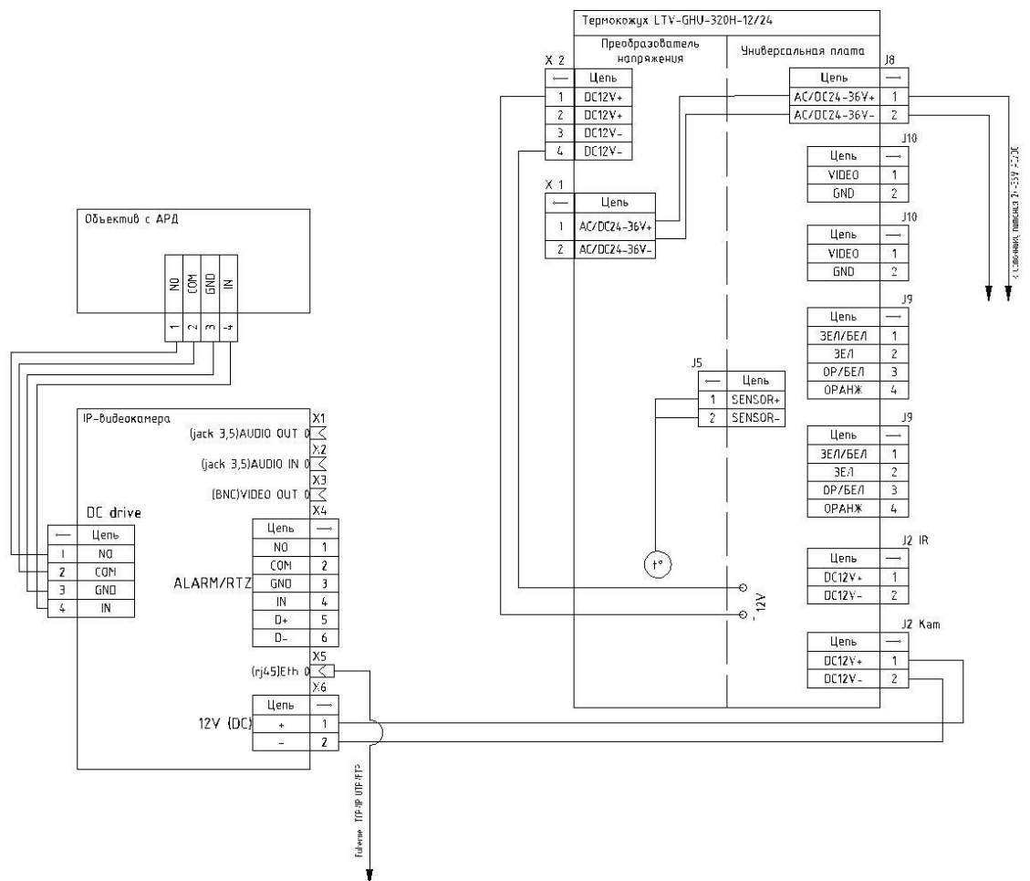
Рисунок 4 – Схема электрических соединений
