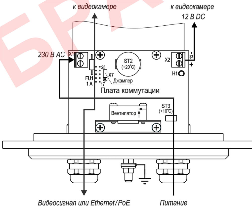
Рисунок 3 – Подключение ТГБ-11-220/12
