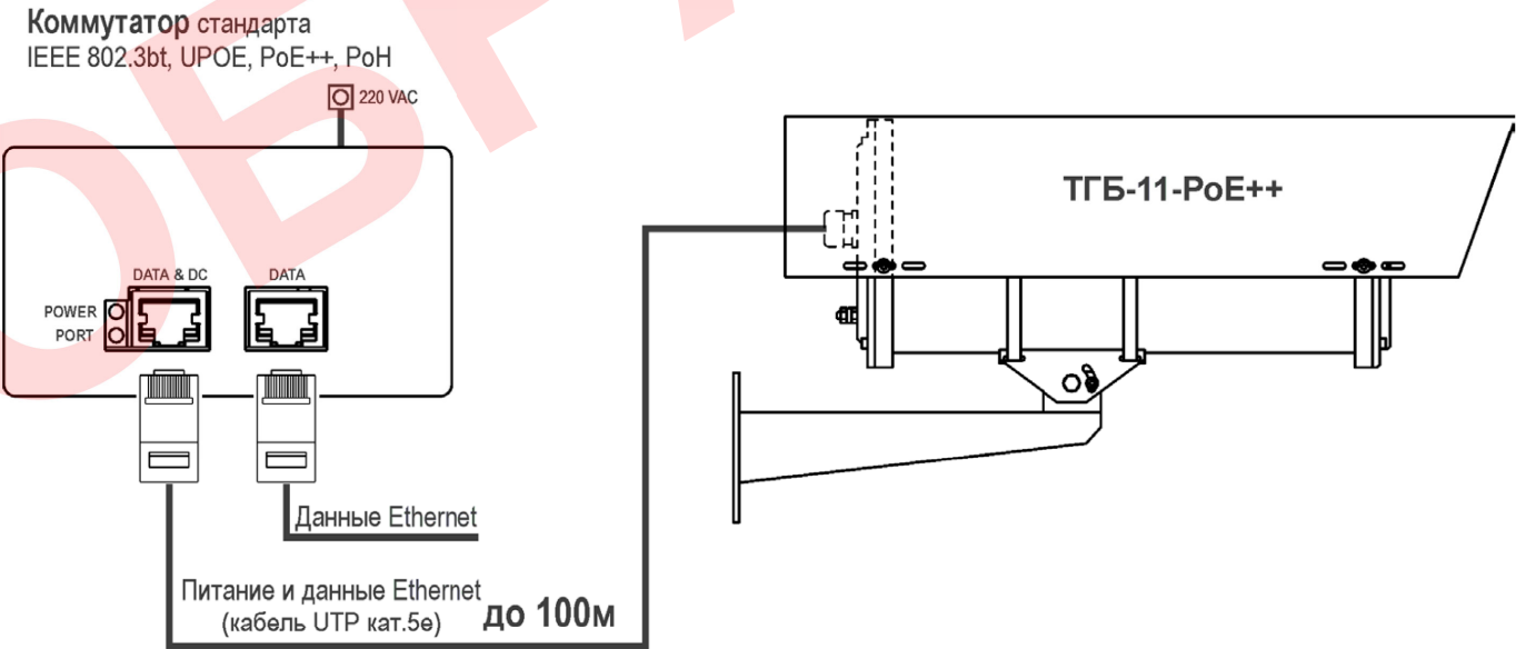
Пример подключения термокожуха ТГБ-11-PoE++
