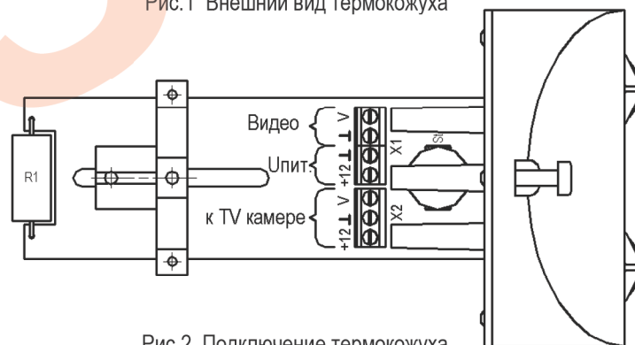
Рис.2 Подключение термокожуха
