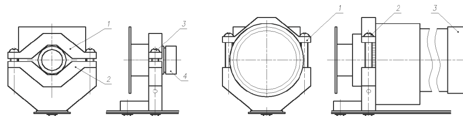
Рис.2 Подключение термокожуха
