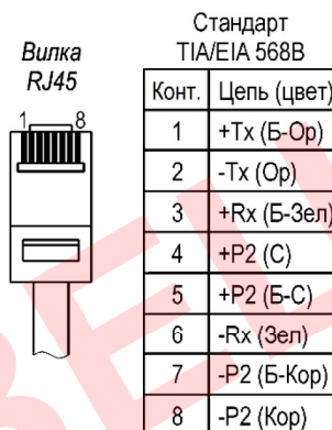
Рисунок 6 – Обжимка вилки RJ45 на кабель кат.5е
