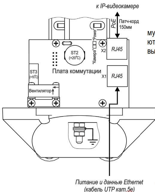
Рисунок 5 – Подключение ТГБ-7-РоЕ+
