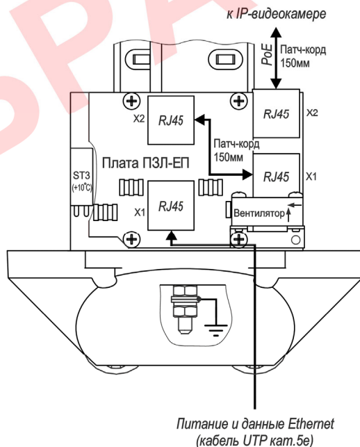
Рисунок 7 – Подключение ТГБ-7-РоЕ+ с платой ПЗЛ-ЕП
