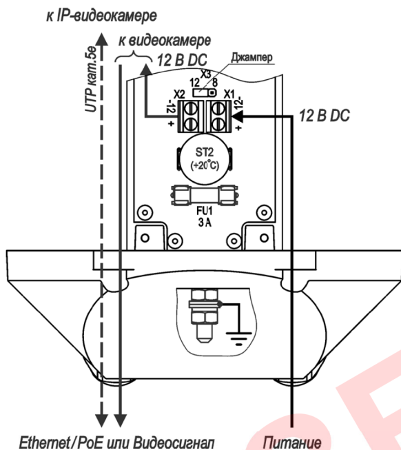
Рисунок 9 – Подключение ТГБ-7С-12
