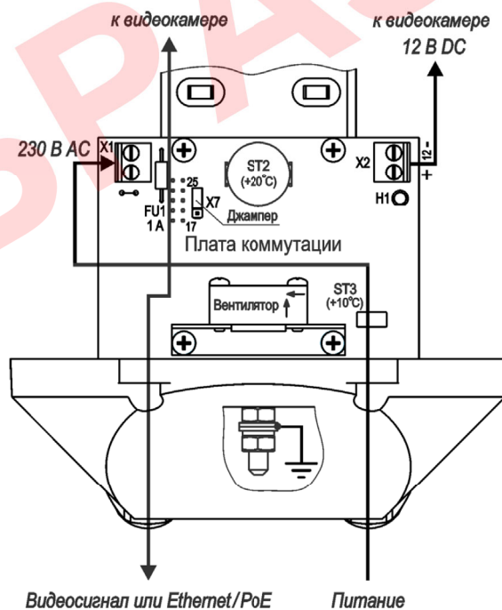
Рисунок 4 – Подключение ТГБ-7С-220/12
