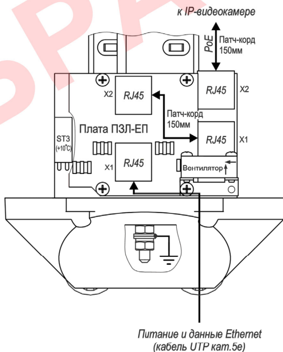
Рисунок 7 – Подключение ТГБ-7С-PoE+ с платой ПЗЛ-ЕП
