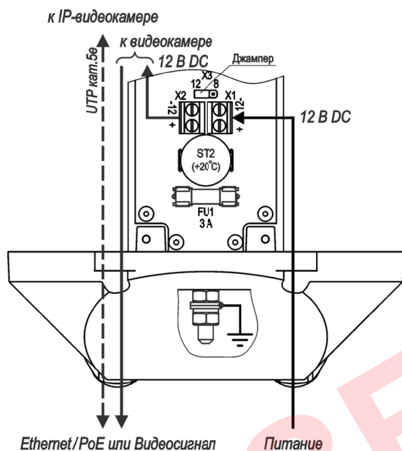
Рисунок 9 – Подключение ТГБ-7С-12
