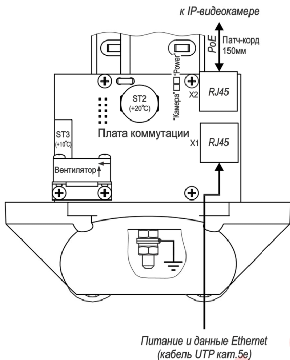
Рисунок 5 – Подключение ТГБ-7С-PoE+
