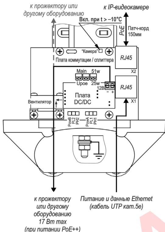
Рисунок 8 – Подключение ТГБ-7У-PoE++
