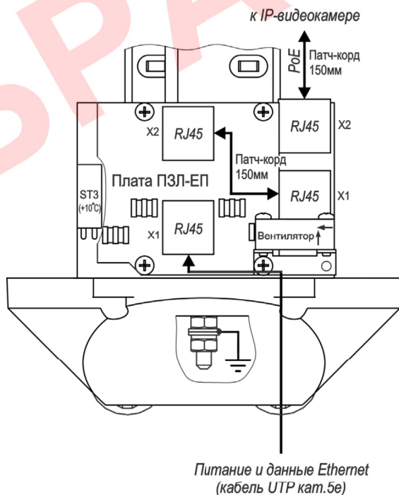
Рисунок 7 – Подключение ТГБ-7У-PoE+ с платой ПЗЛ-ЕП
