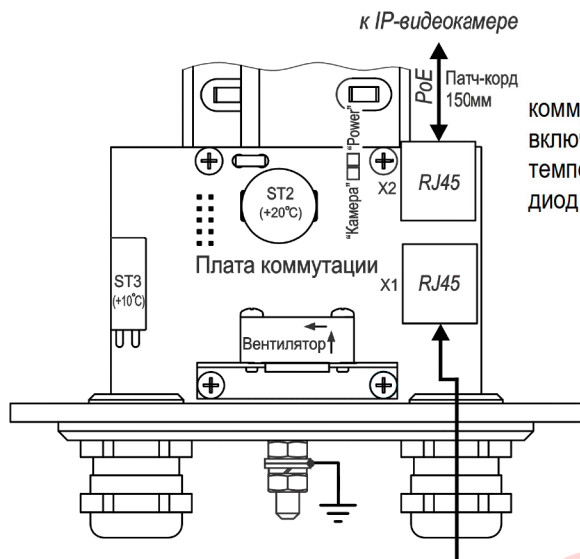
Вилка RJ45
