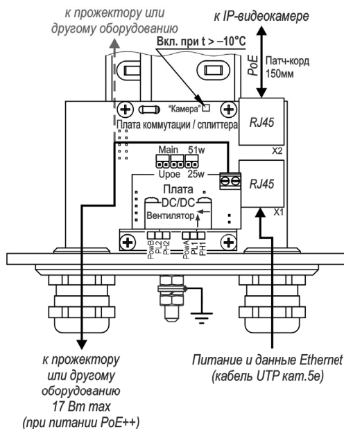
Рисунок 8 – Подключение ТГБ-9У-РоЕ++
