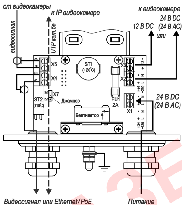
Рисунок 3 – Подключение ТГБ-9У-24/12
