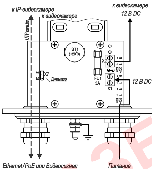
Рисунок 9 – Подключение ТГБ-9У-12
