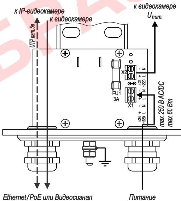
Рисунок 10 – Подключение ТГБ-9У (без обогрева)
