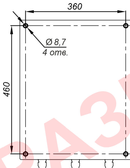
Рисунок 5 – Расположение и габариты отверстий для крепления термощафа к стене
