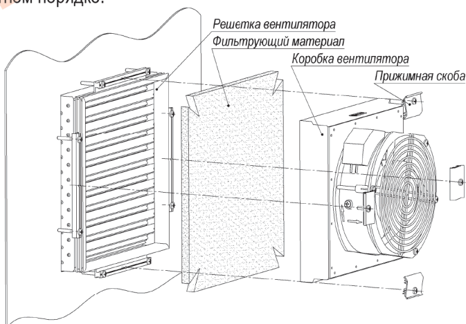
Рисунок 4 – Замена фильтрующего материала
