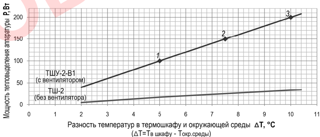
График 1 – Зависимость мощности тепловыделения устанавливаемой в термощаф аппаратуры от разности температур в термощафу и окружающей среды
