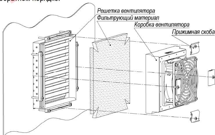
Рисунок 4 – Замена фильтрующего материала
