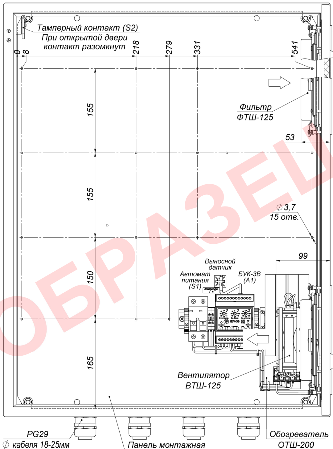
Рисунок 1 – Устройство термошкафа (дверь открыта на 90°, стрелками указано направление воздушного потока)
