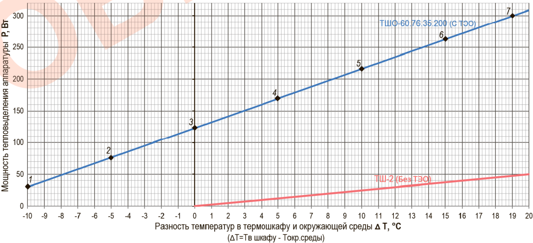
График 1 – Зависимость мощности тепловыделения устанавливаемой в термощаф аппаратуры от разности температур в термощафу и окружающей среды
