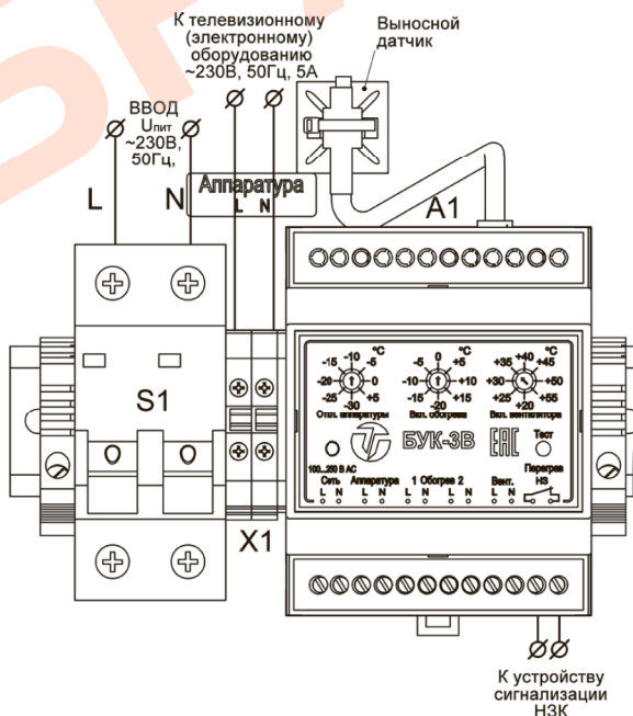
Рисунок 2 – Подключение термощкафа
