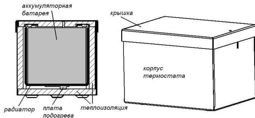
Рис.1 Термостат
