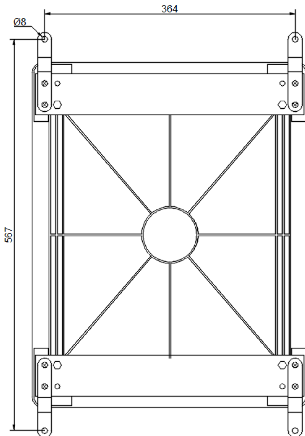
Рисунок 7.2 - Разметка крепления
