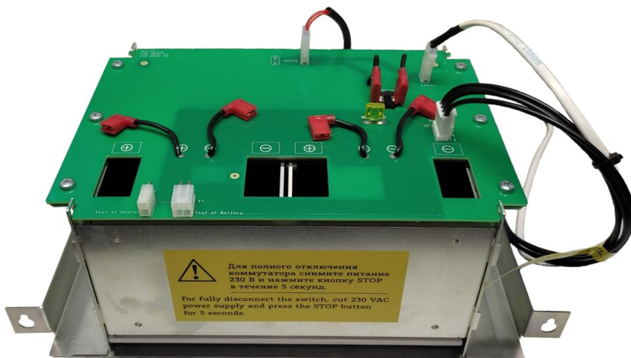
Рисунок 3.6 – отсек АКБ.
