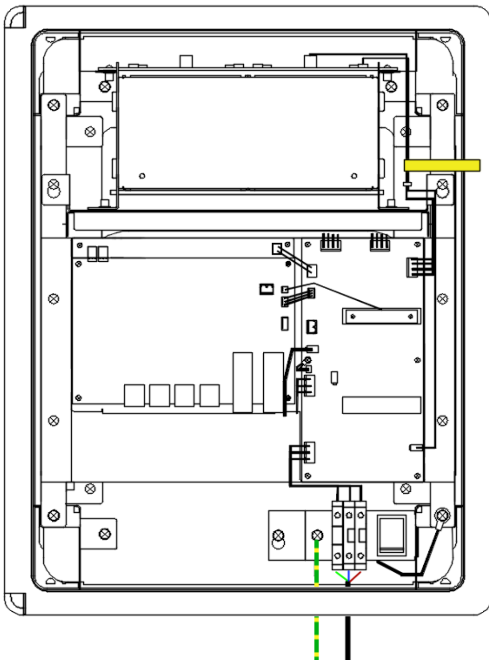
Рисунок 7.7 - Схема подключения коммутатора.
