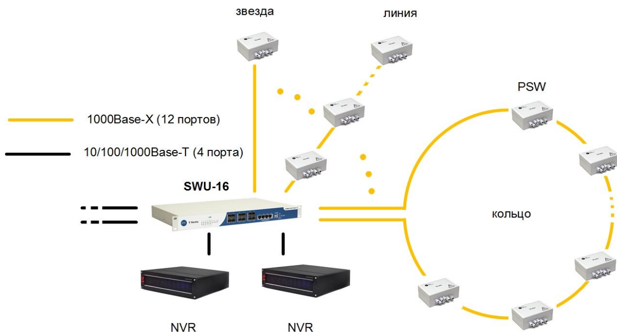
Рисунок 1.1 - Схема подключения
