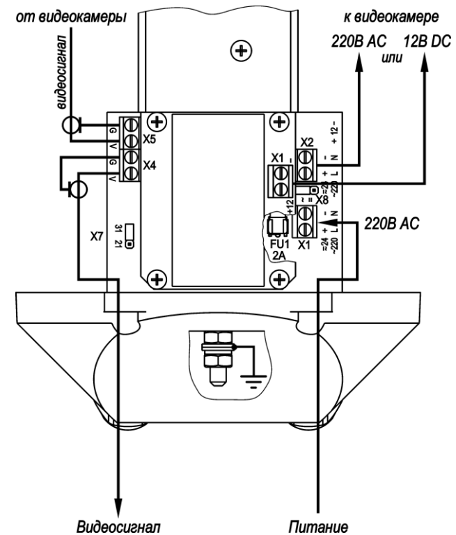
Рис.3 Подключение ТГБ-7У- ~220/12(~220)
