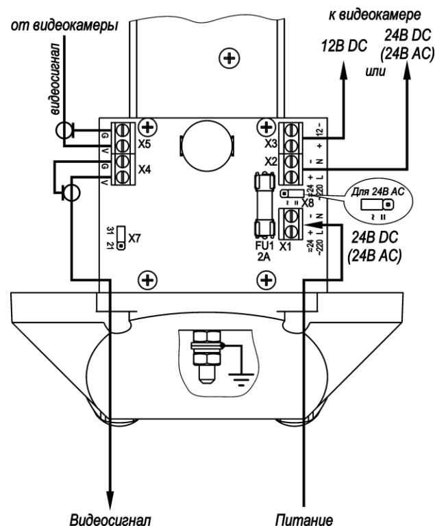
Рис.2 Подключение ТГБ-7У-24/12(24); ~24/12(~24)
