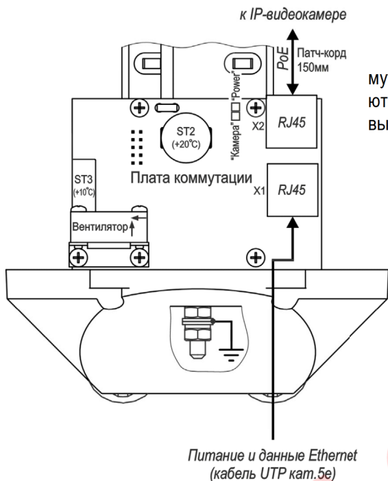
Рисунок 5 – Подключение ТГБ-7У-PoE+
