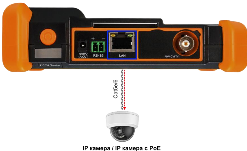
Рис. 10 Подключение IP-видеокамеры (в том числе с PoE питанием)
