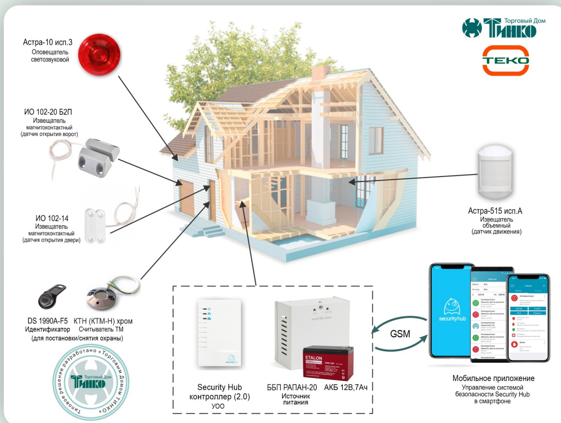
Автономная проводная система охранной сигнализации на базе контроллера Security Hub для дома, дачи, коттеджа
