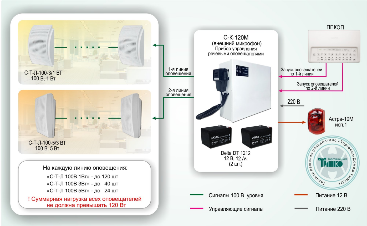
Схема построения системы оповещения о пожаре
