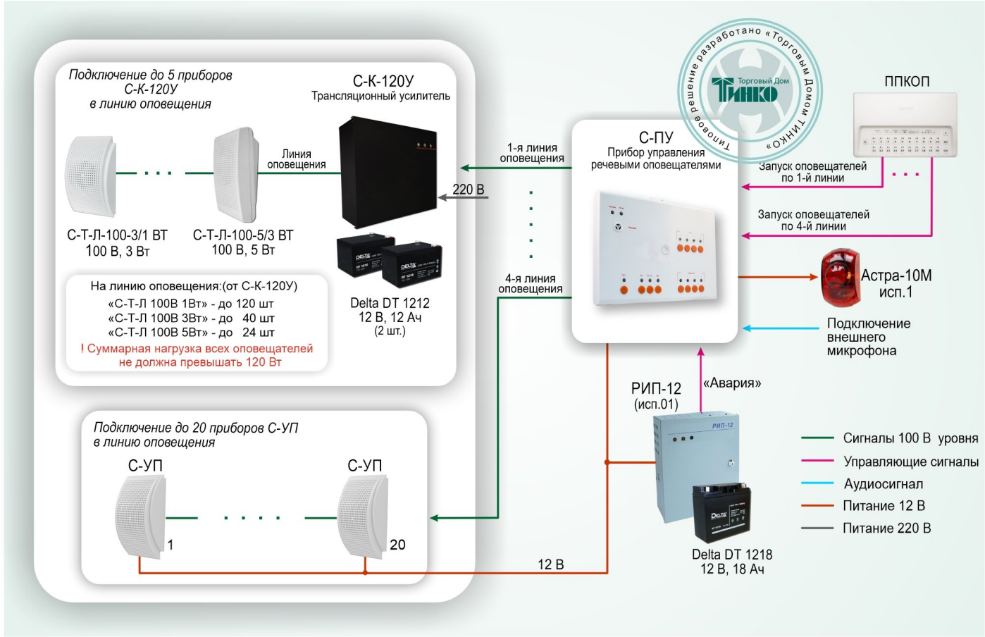
Схема построения системы оповещения о пожаре
