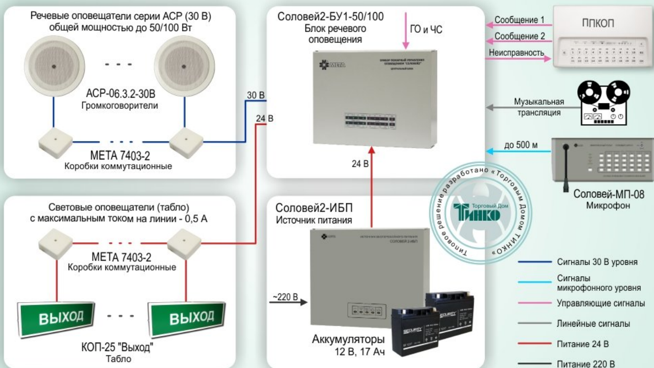
Однозонная СОУЭ 3-го типа (50 / 100 Вт)
