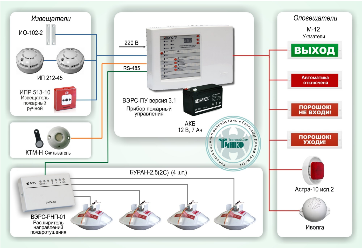
Схема построения системы пожаротушения на основе "ВЭРС-ПУ версия 3.1"
