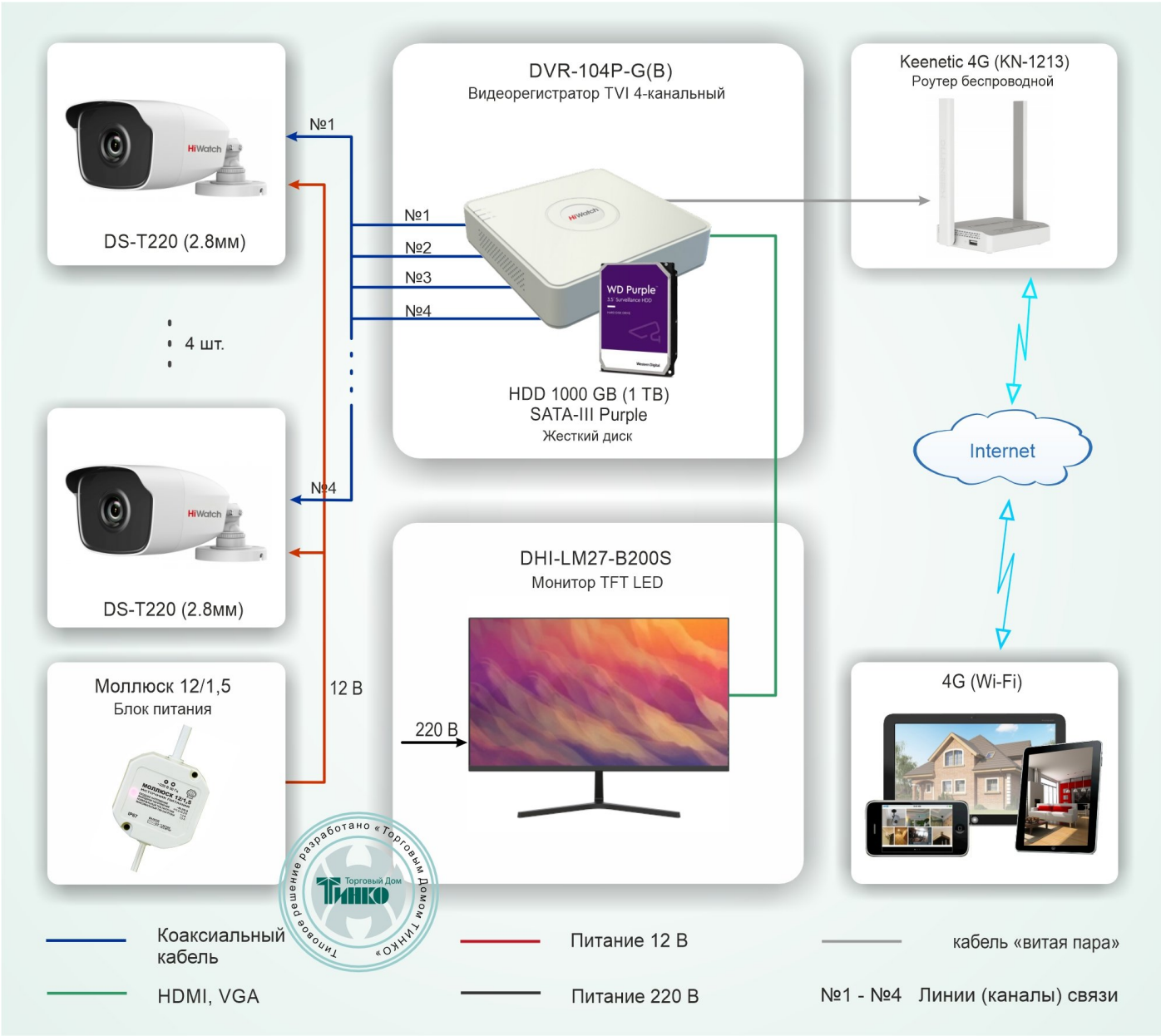
Схема построения системы видеонаблюдения за периметром дачи
