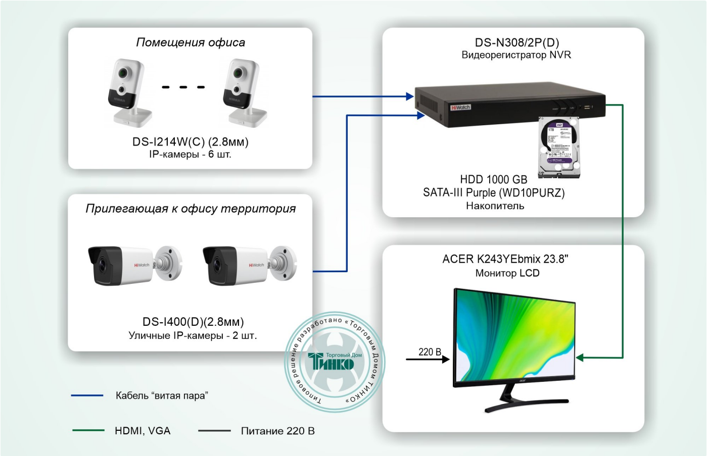
Схема построения системы IP-видеонаблюдения для офиса
