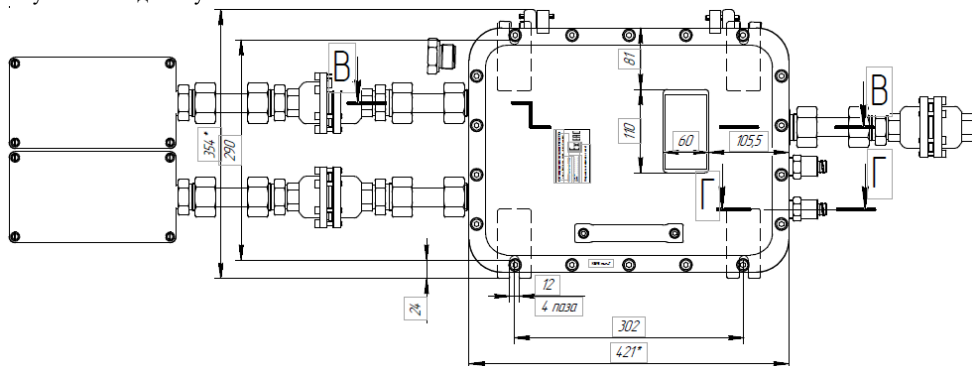
Рисунок 2 – Вид сверху.
