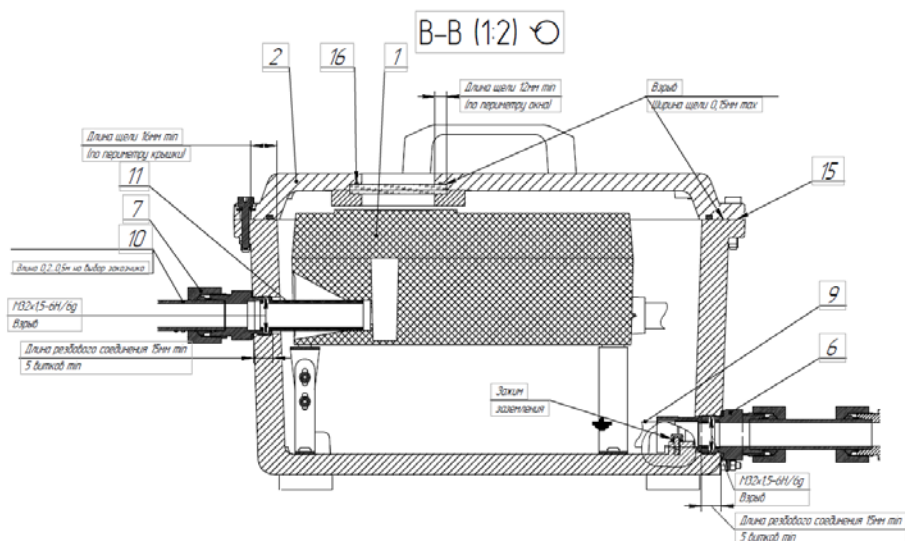
Рисунок 6 – Разрез В-В.
