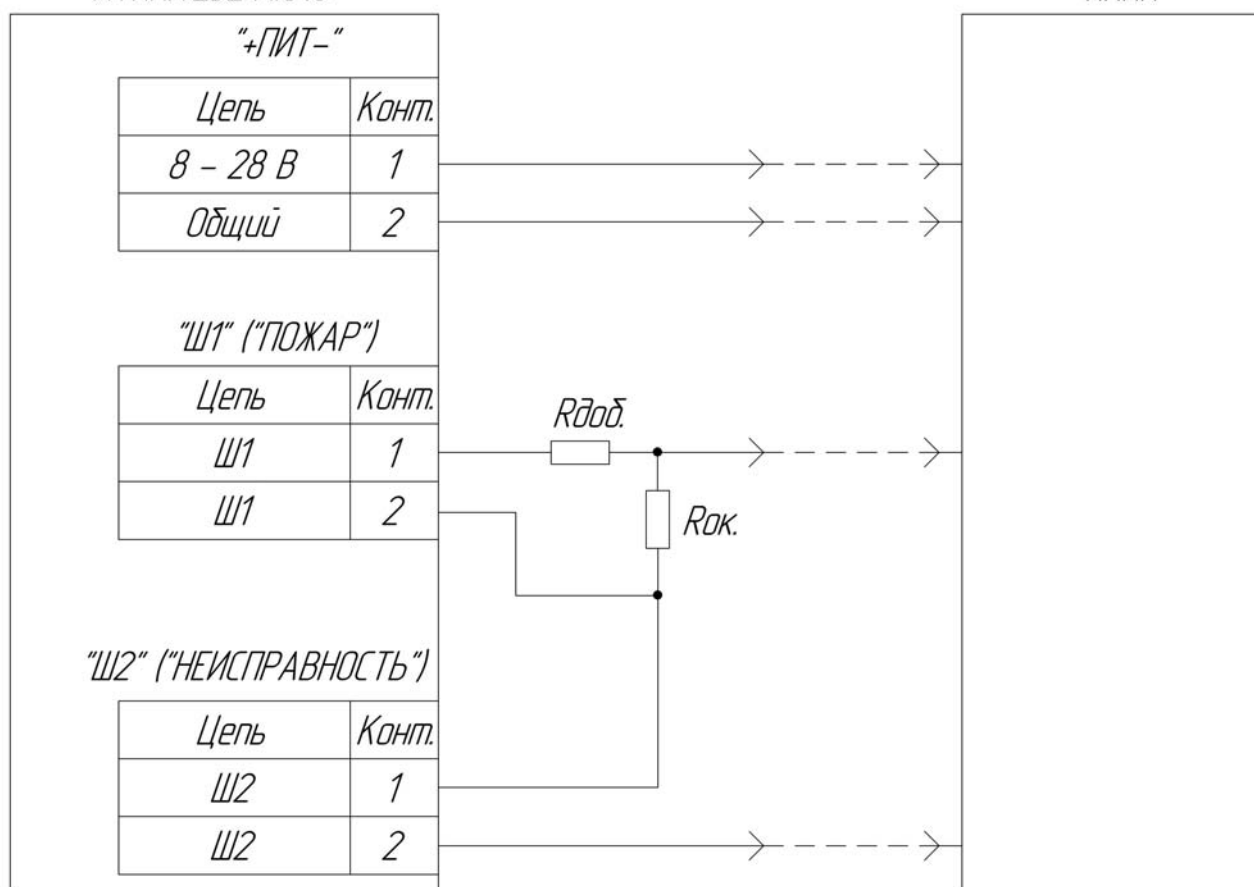
Рисунок А.1 – Схема подключения изделия по 4-х проводному шлейфу
