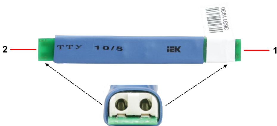
Рис.2 Датчик TMS-SL, разъемы
