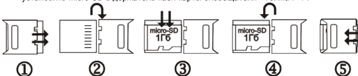
Рис. 5. Установка micro-SD в держатель карты оповещателя "Толмач"-F
