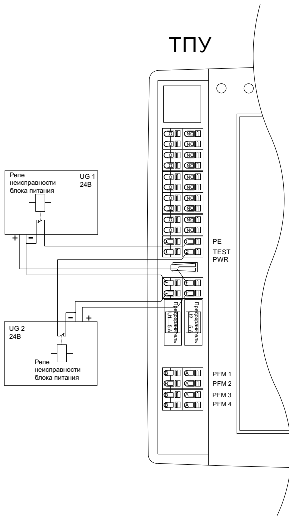
Рисунок 9 – Схема подключения с двумя источниками и выходом контроля исправности блока питания типа «сухой контакт»
