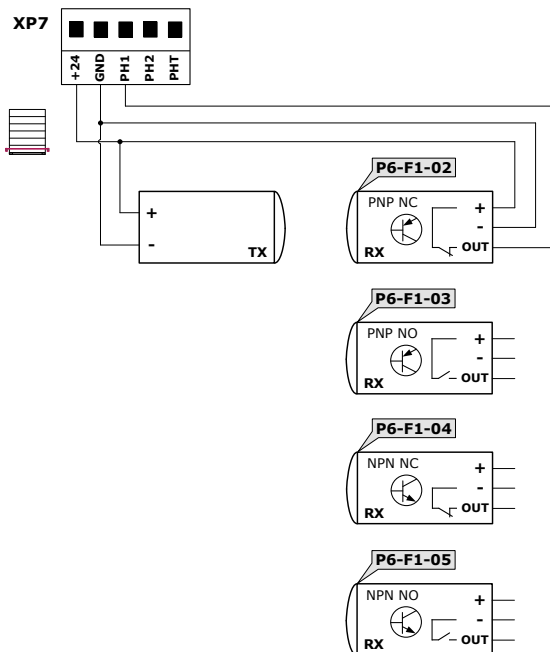
Фотоэлементы с транзисторным выходом разного типа
