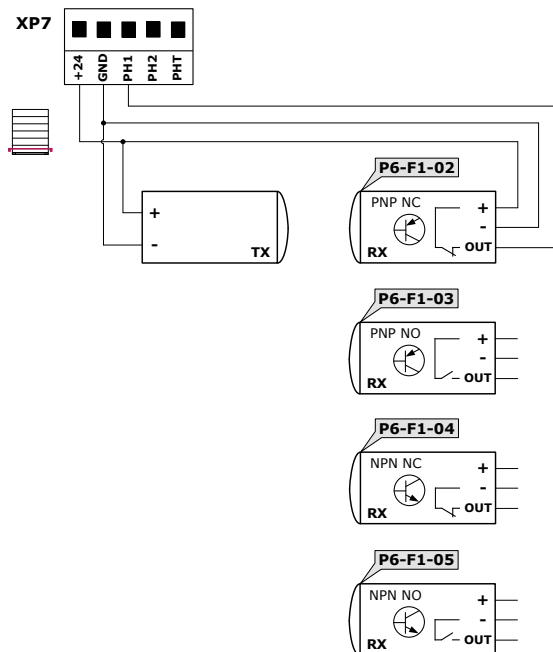
Photocellules avec différents types de sortie transistor
