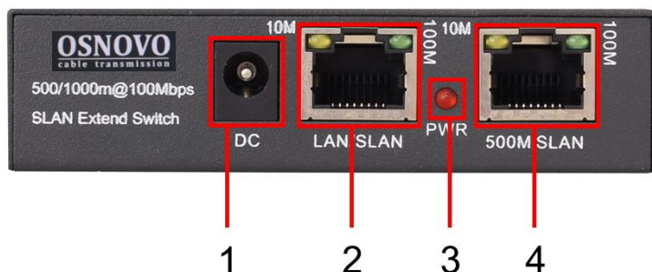
Рис. 2 Панель подключения удлинителя TR-IP1(800м)
