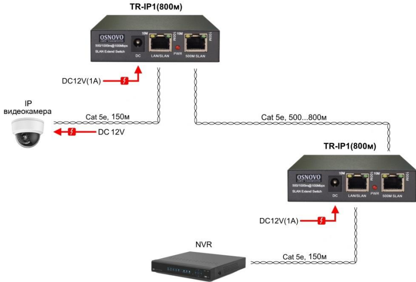
Рис.3 Типовая схема подключения удлинителя TR-IP1(800м)
