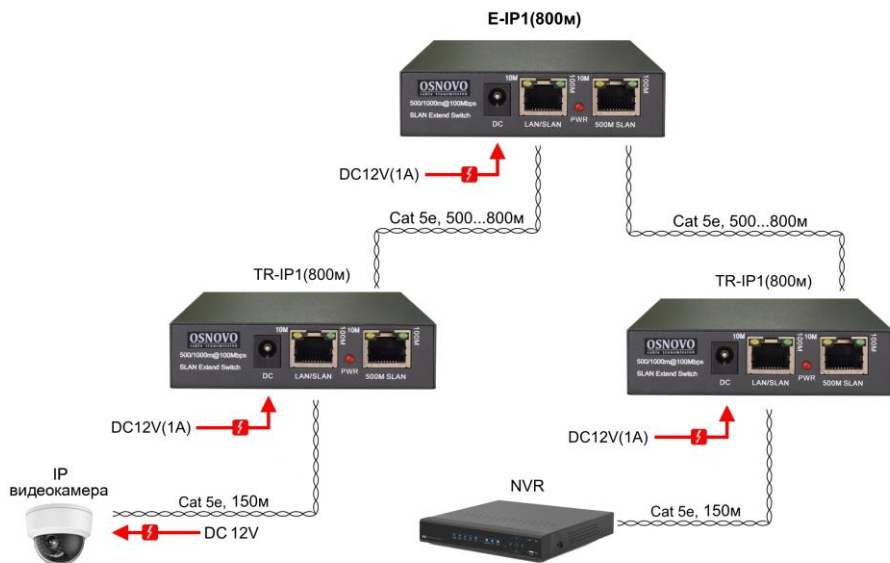
Рис.4 Схема подключения удлинителей TR-IP1(800м) и E-IP1(800м)
