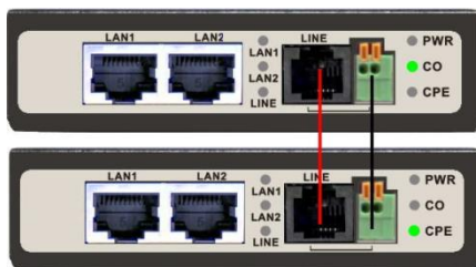
Рис. 8 Прямое соединение CO (сервера) и CPE (клиента).
