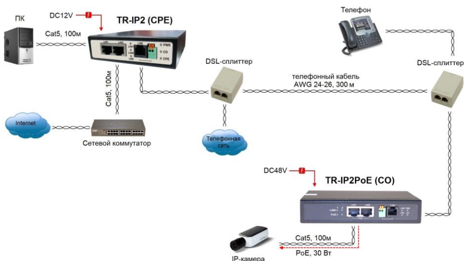
Рис. 7b Схема подключения TR-IP2PoE (CO) и TR-IP2 (CPE) для организации IP-видеонаблюдения с параллельным подключением телефонного аппарата
