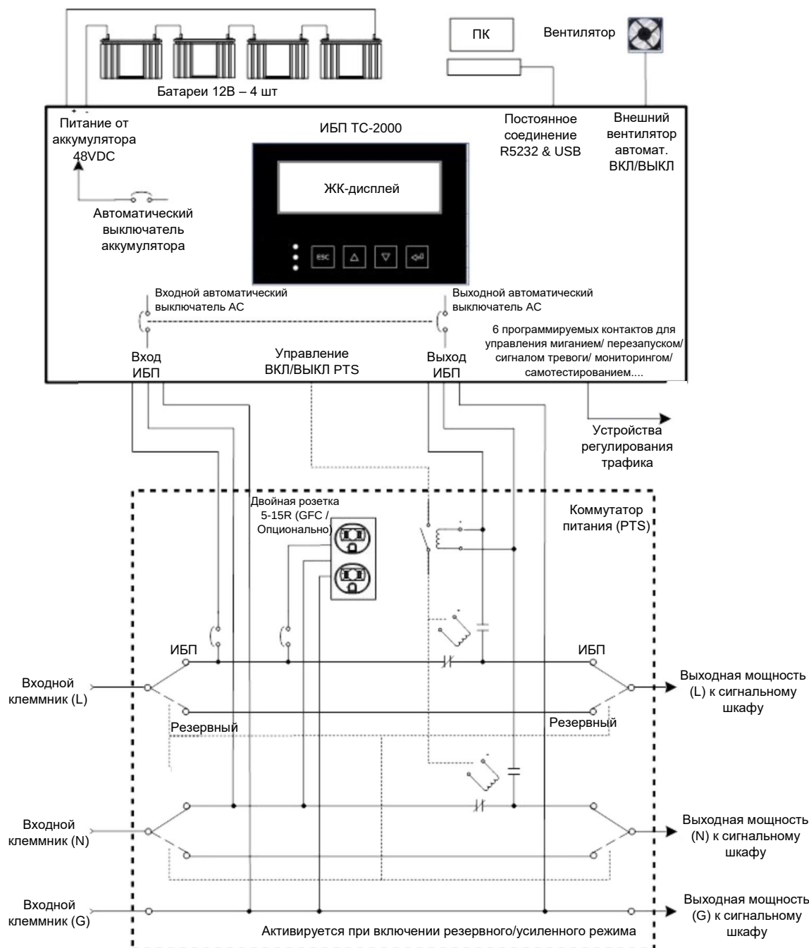
Рисунок 1 Упрощенная блок-схема системы ИБП ТС 120V
