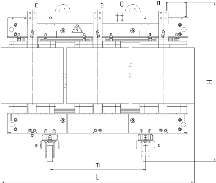
Рисунок А.1 – Габаритные размеры OptiTrans D TS(D)L(L) 10 (20, 35) кВ
