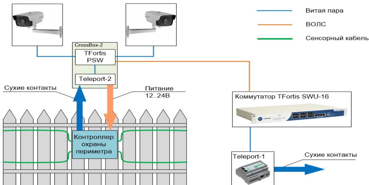
Рис. 5.3.1.3. структура системы
