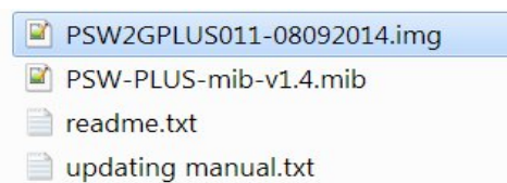
Рис. 5.3.20.1. Файл *.img
