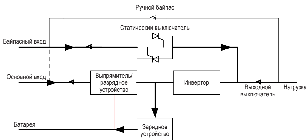
Рис. 2-3. Схема работы в режиме работы от батареи
