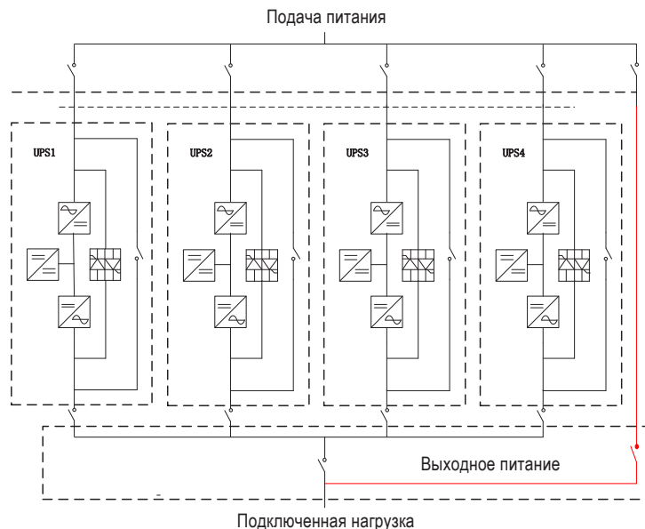
Рис. 5-5. Параллельная схема
