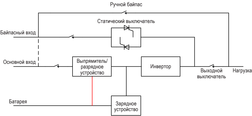
Рис. 2-1. Конфигурация ИБП
