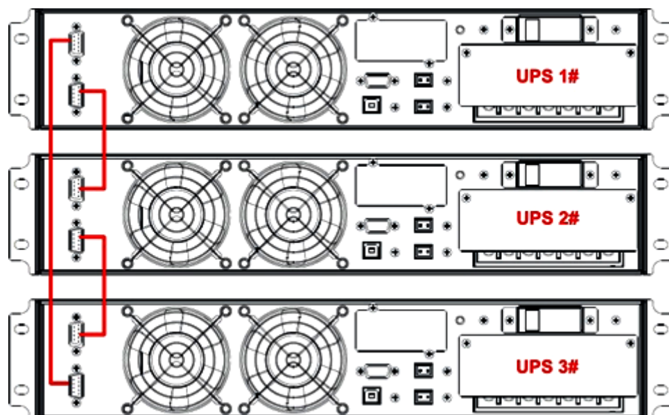
Рис. 28. Подключение портов при 3 ИБП (6 кВА, 10 кВА) в параллель
