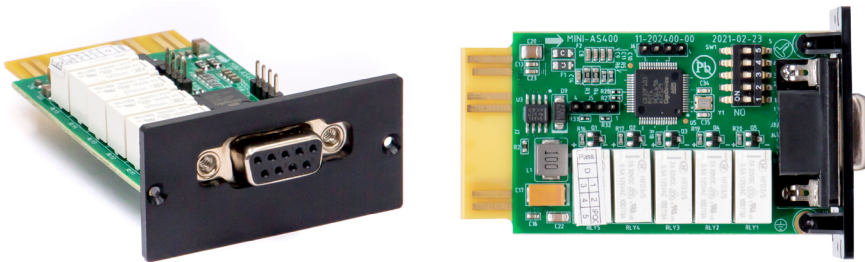
Рис. 23. Внешний вид платы DRYCONTM
