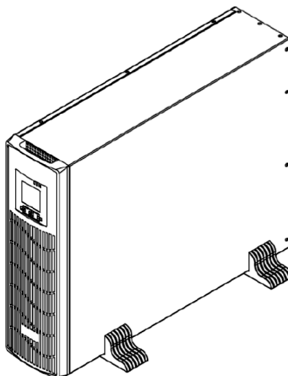
Рис. 12. Вертикальная установка ИБП серии Trio TM (TRIOTM15AOP, TRIOTM20AOP)
