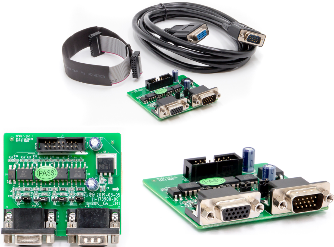
Рис. 25 Внешний вид платы параллельной работы (PARTM)
