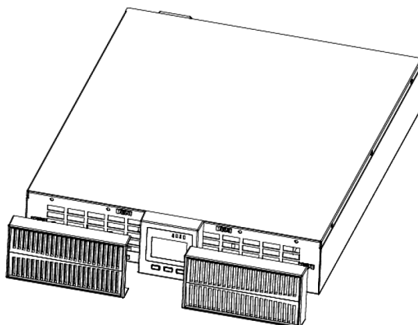
Рис. 13. Снятие защитных крышек с ИБП (только для моделей TRIOTM6AOP, TRIOTM10AOP). Поверните дисплей, как показано на рис. 14.
