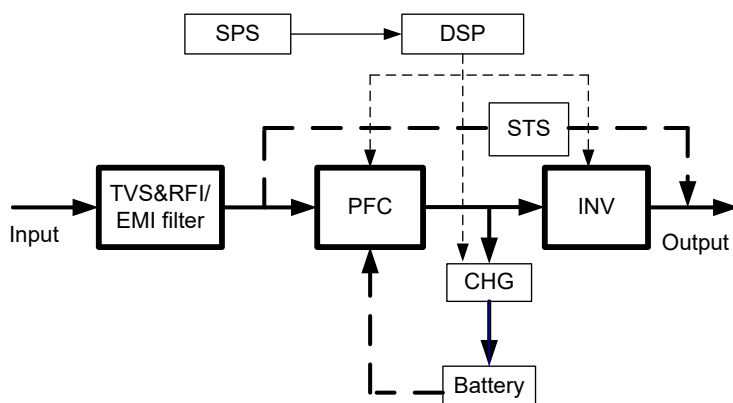
Рис. 3. Блок-схема
