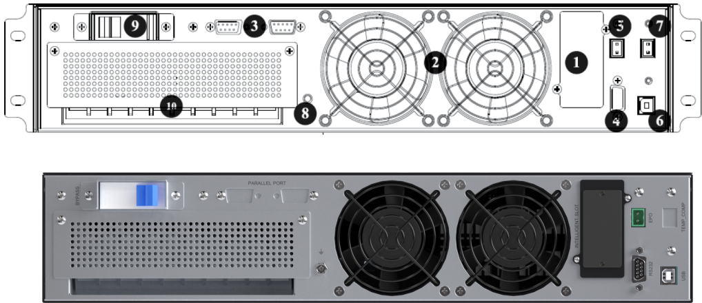
Рис. 17. Задняя панель ИБП Trio TM (TRIOTM6A0P, TRIOTM10A0P)
