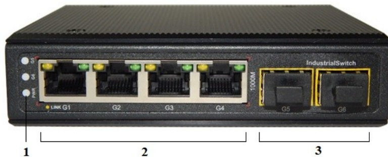
Рисунок 1 - Передняя панель коммутатора.
