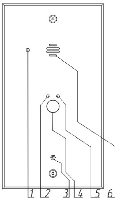
Рисунок 25 - «Тромбон IP-ВП исполнение В», вид спереди.
