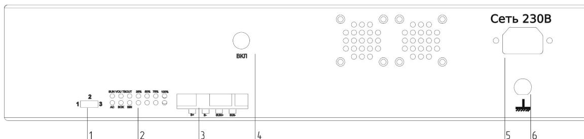
Рисунок 31 - «Тромбон IP-K-8-AKB», вид сзади..
