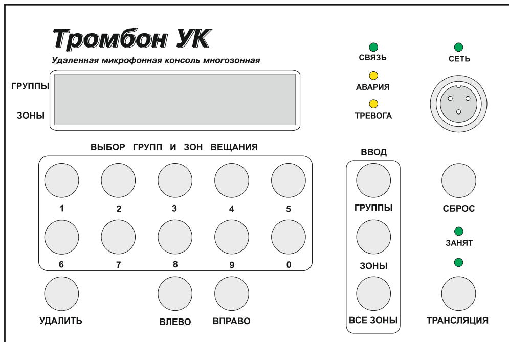
Рисунок 3 – Внешний вид удалённой консоли «Тромбон УК».
