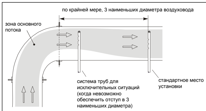
Рис. 4.20: Распределение потока в канале без дефлекторов
