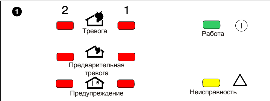
Рис. 2.6: Индикация TITANUS® (пояснения см. № 1 в таблице на следующей странице)
