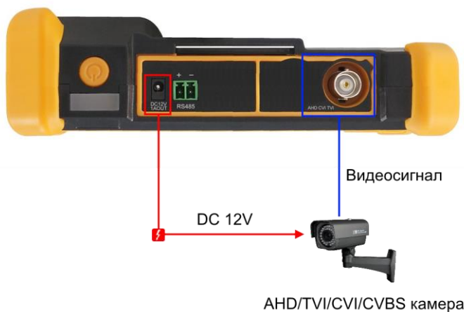
Рис. 9 Подключение AHD/TVI/CVI/CVBS видеокамеры к тестеру
