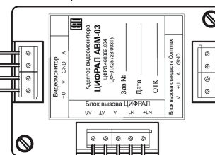
Адаптер видеомонитора с гальваноразвязкой ЦИФРАЛ АВМ-03
