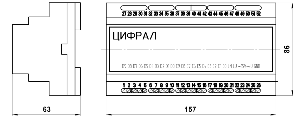
Рисунок Г.2 Габаритные и установочные размеры коммутатора ЦИФРАЛ КМГ-100.1
